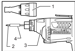
1. Локатор 2. Бита 3. Корпус редуктора 4. Магнитный держатель бит
